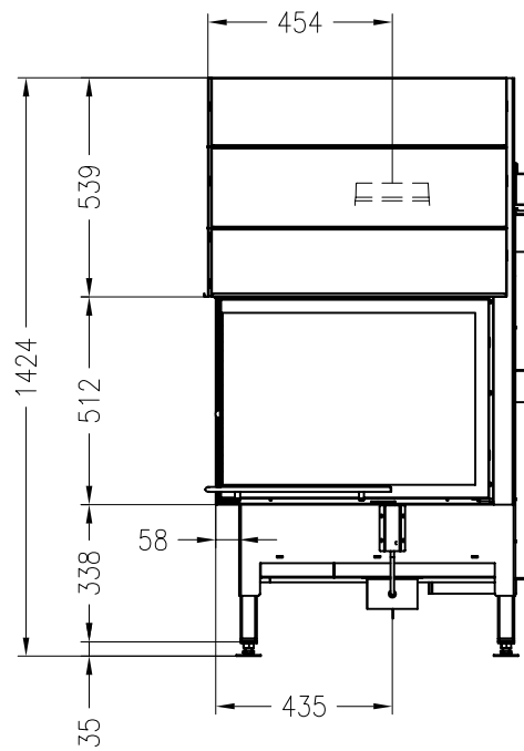
Vorderansicht M~1:20
