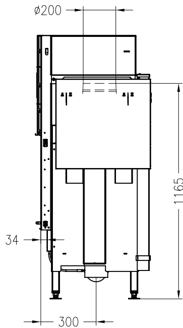
Seitenansicht M~1:20
