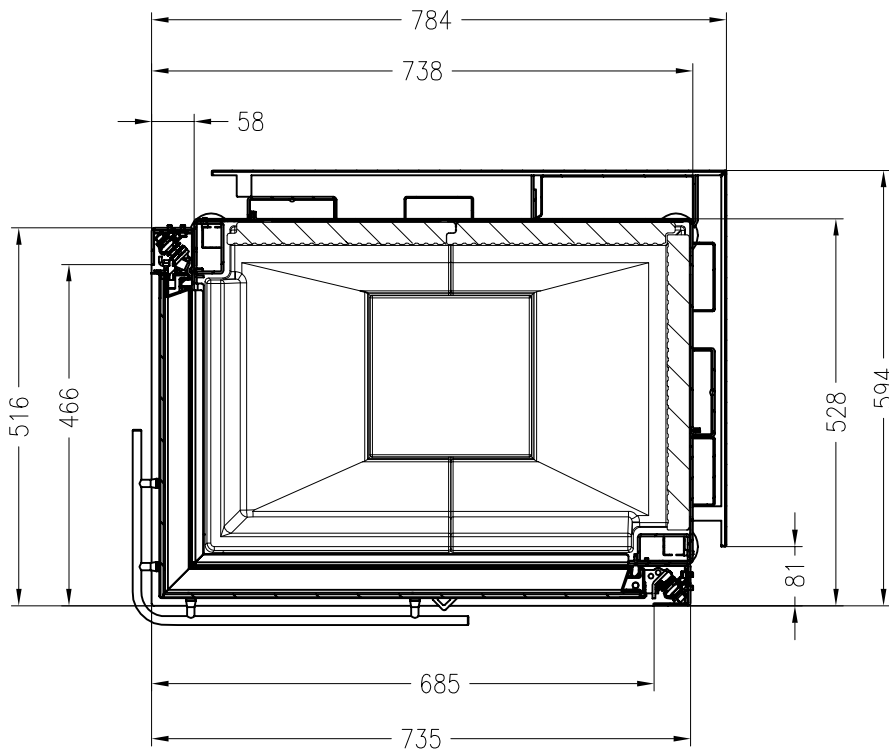
Horizontalschnitt M~1:10
