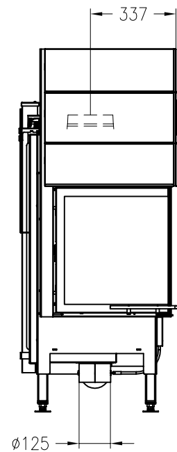
Seitenansicht M~1:20
